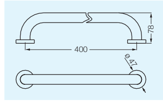
0715.10.1/37 Agarradera para bañera de 40 cm.
