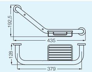
0714.10/37 Agarradera angular con jabonera.
