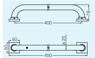
0715.10.2/37 Agarradera para bañera de 40 cm.
